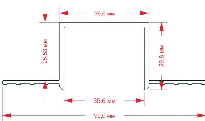
PL-4100 универсальный профиль под шпаклевку
